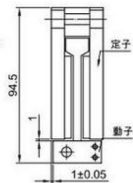
動、定子組合圖
