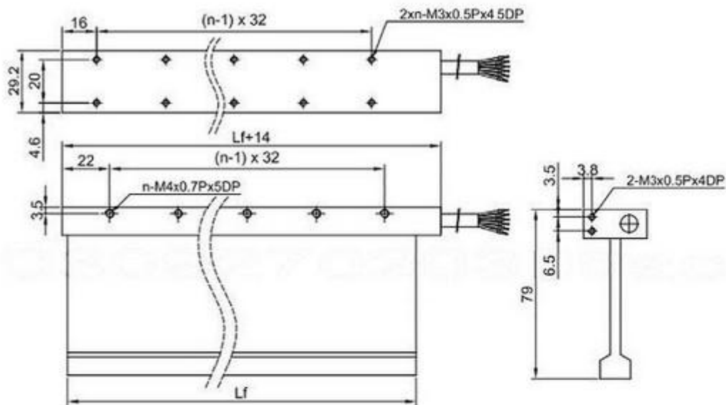
定子尺寸圖
