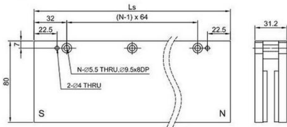
定子尺寸圖
